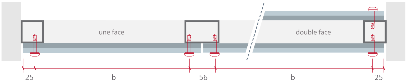
Plan d'Élévation
